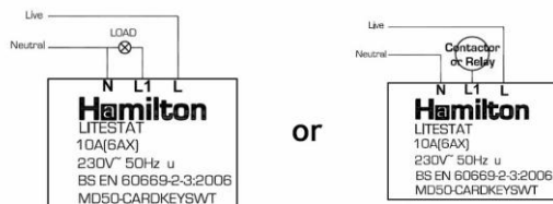
Wiring
